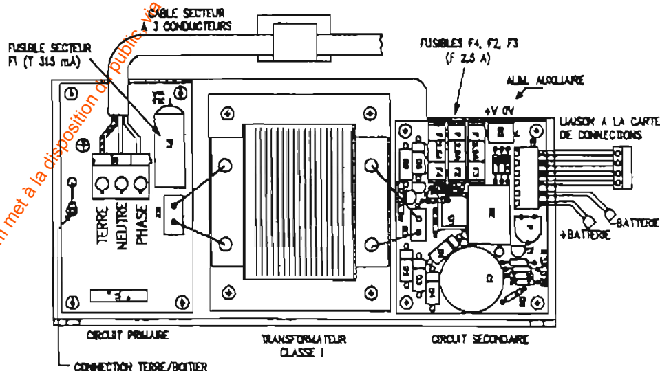
Figure 2-1 : Présentation du module chargeur
