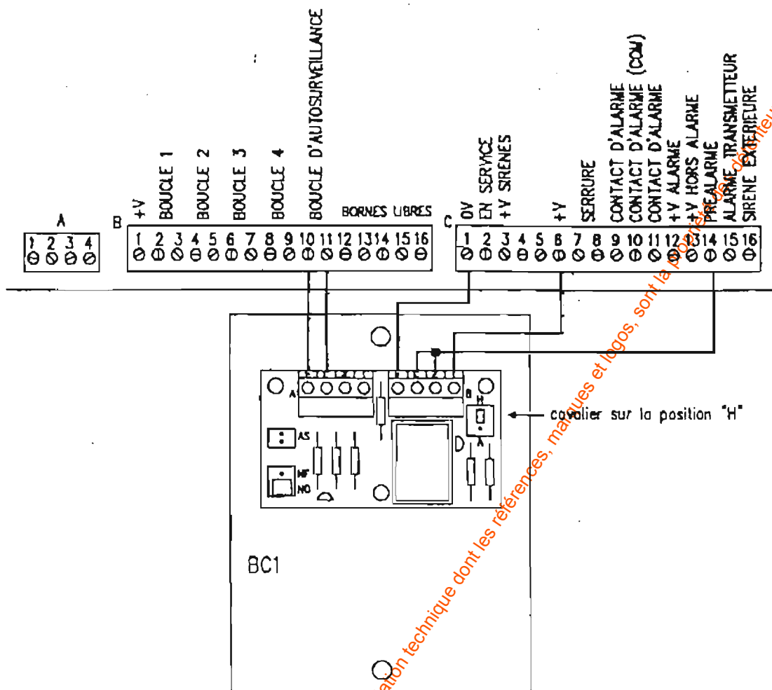
Schéma de raccordement entre la centrale d'alarme ARENA et le boîtier BC1.
