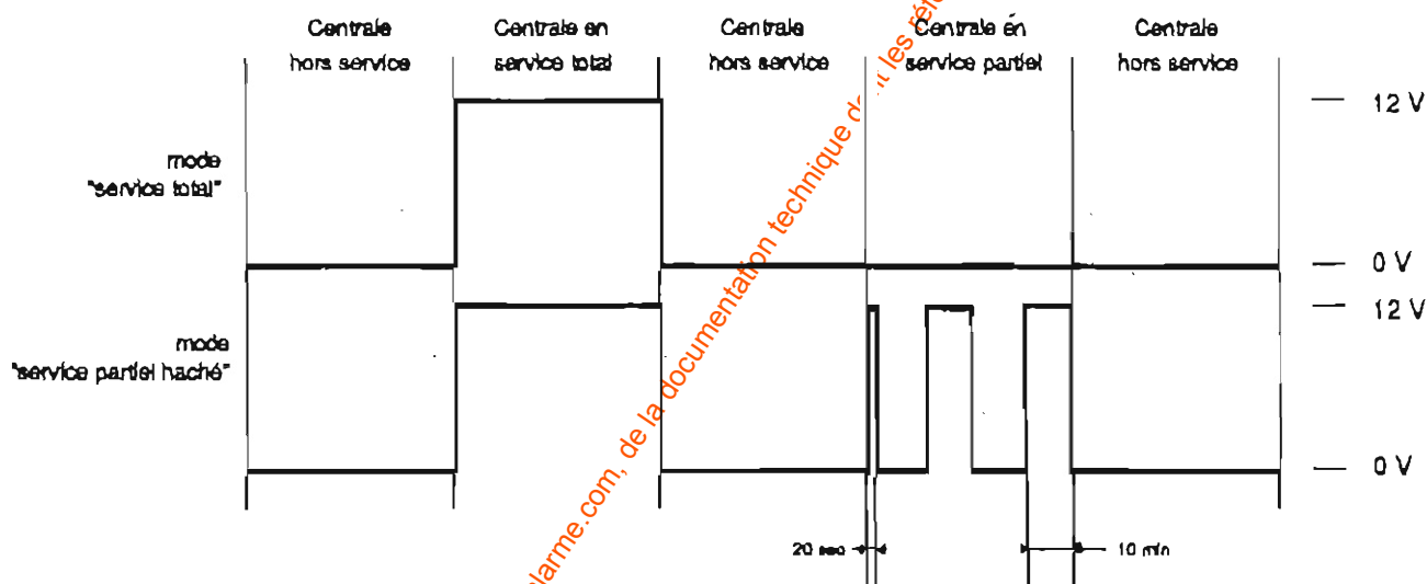
Diagramme des modes d'activation de la sortie «+V EN SERVICE TOTAL»
