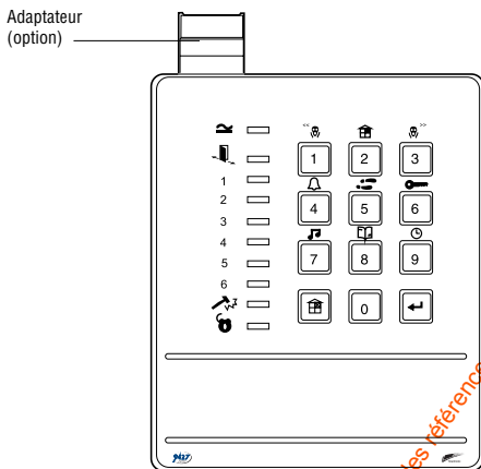
Figure 2. Clavier déporté 9427
