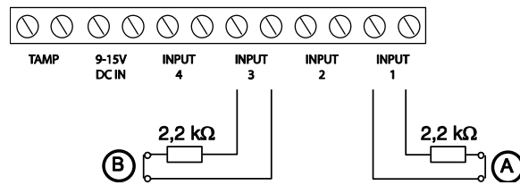
Figure 5. Raccordement de résistances de fin de ligne
