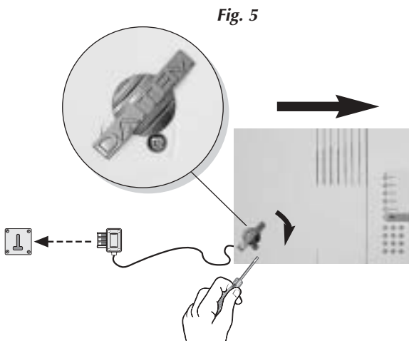
Encoches de passage de câble
