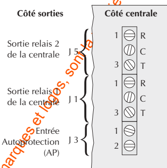
Caractéristiques électriques du bornier de raccordement
